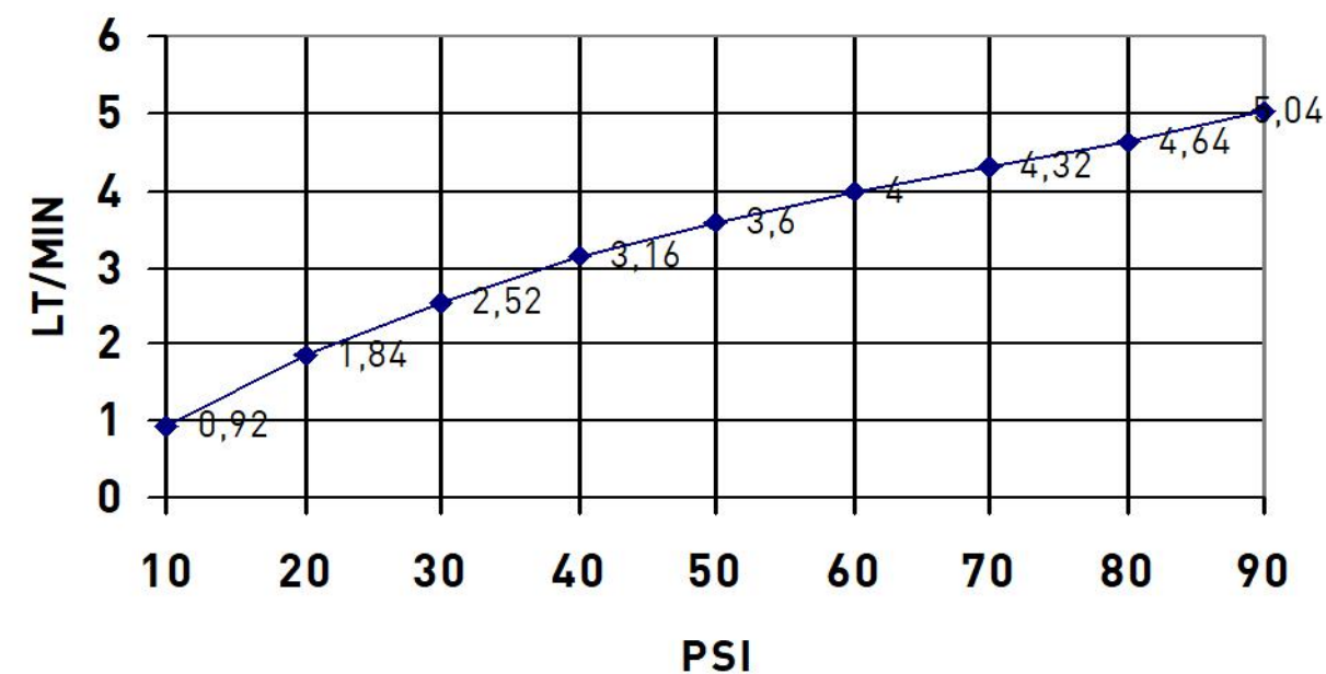
GRAFICO PORTATA / FLOW RATE
